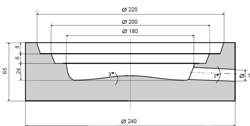
KONDENZÁTNÍ JÍMKA KJ DN 180/200 hmotnost 3,7kg
