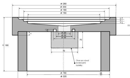
KONDENZÁTNÍ ZÁKLADOVÁ JÍMKA UNIVERZÁLNÍ KZR DN 160/180/200
